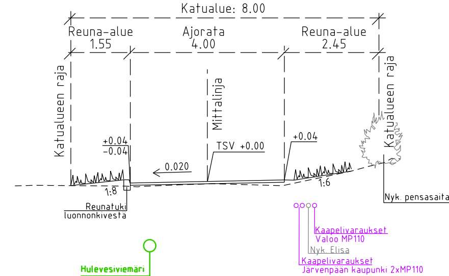
Humalakuja Tyyppipoikkileikkaus plv 7-85, 159-195 (pl 50) 1:100
