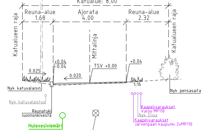
Humalakuja Tyyppipoikkileikkaus plv 93-151 (pl 130) 1:100
